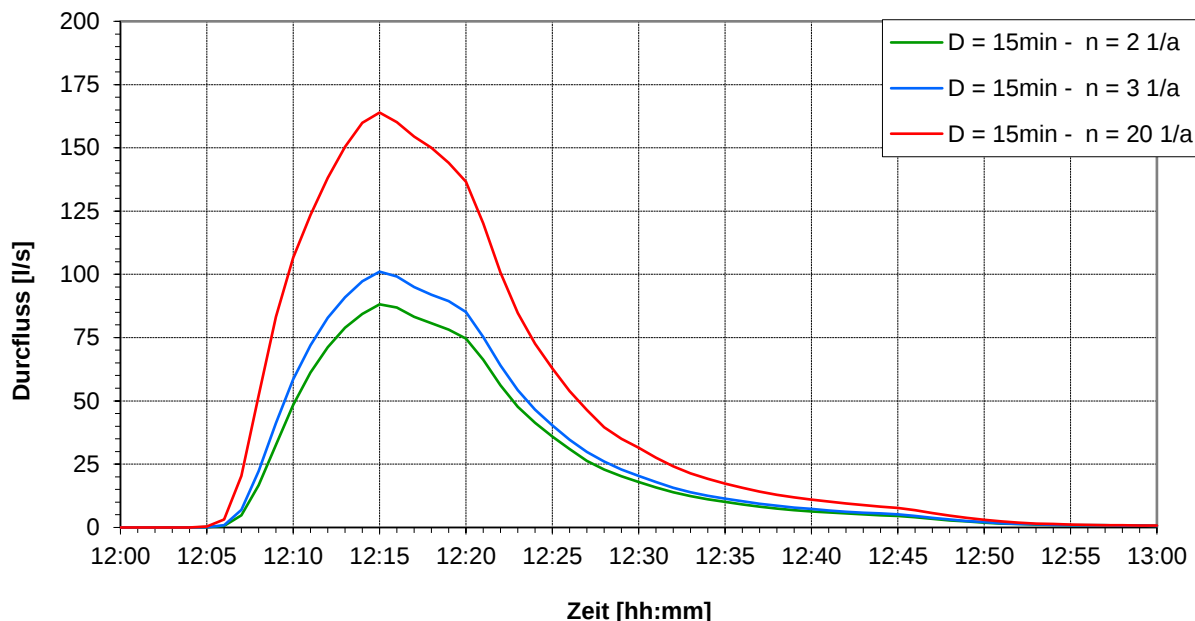
Abbildung Abfluss Baugebiet (Haltung 2.12)
