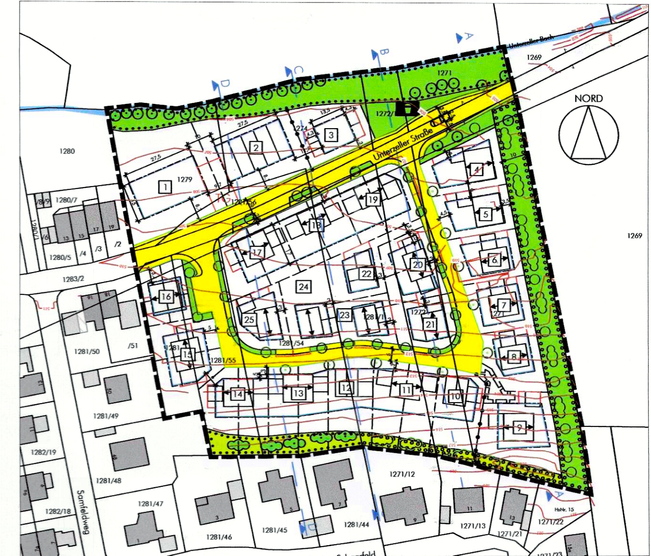
Übersichtsplan, maßstablos
