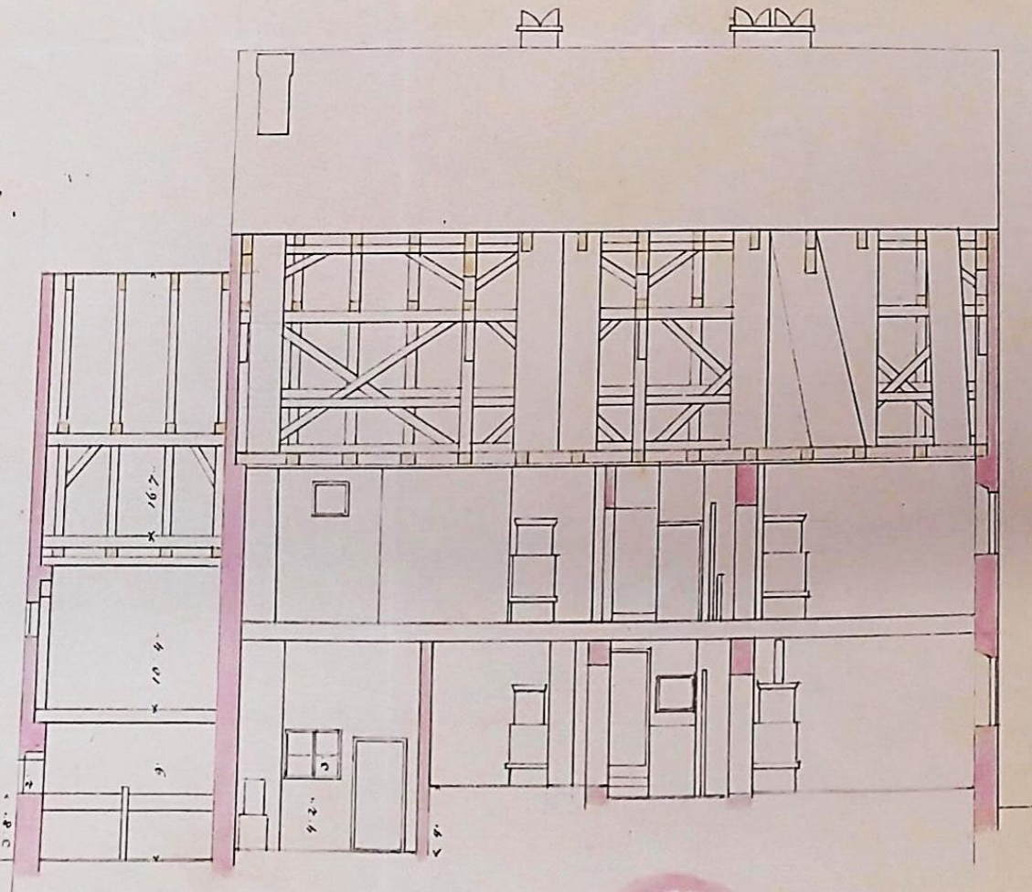
Längenschnitt C.D.
