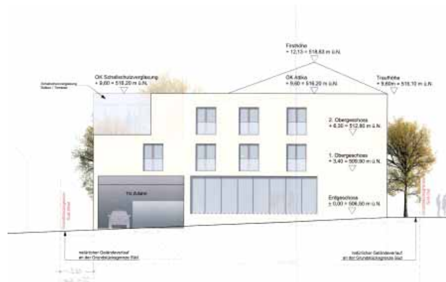
ANSICHT SÜD
