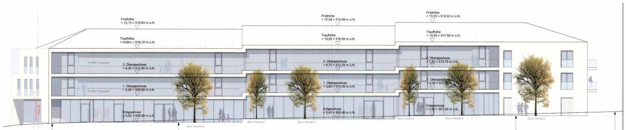
Ansicht Ost
